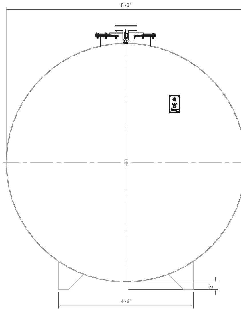
END ELEVATION
