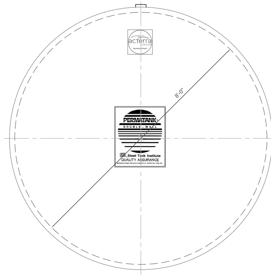
END ELEVATION
