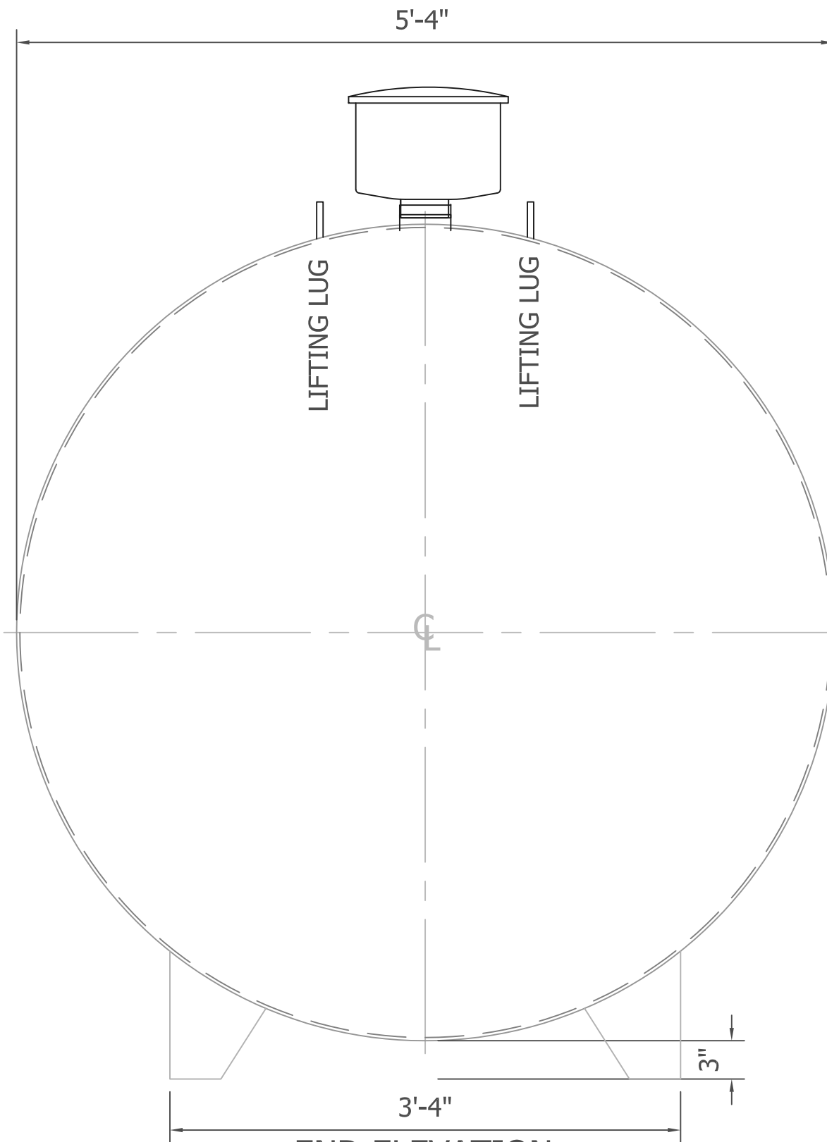
END ELEVATION
